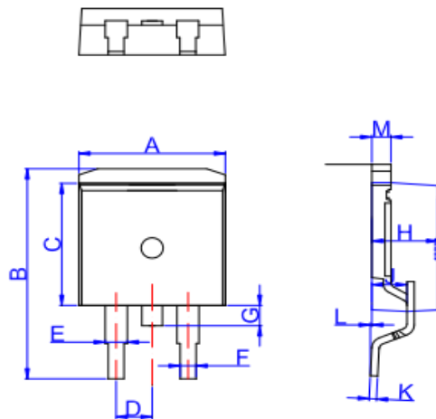
TO-263
